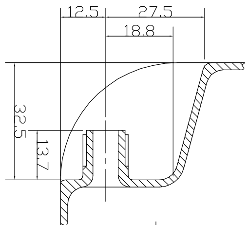
ドリン抜き詳細 S=1:4
