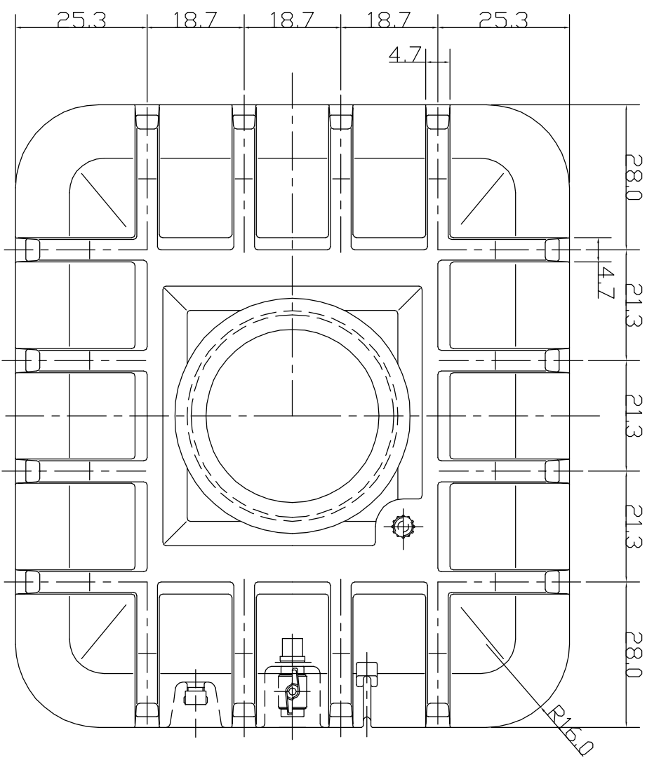
平面図
