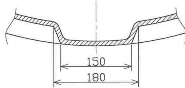
A-A断面
