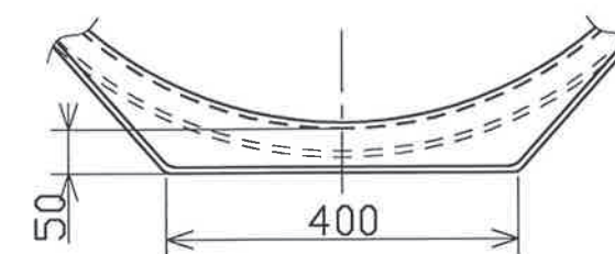
A・B部断面図
