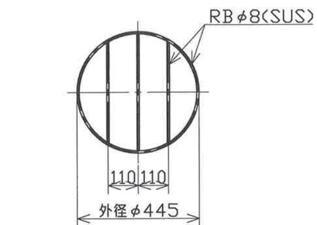
落下防止金具（オプション）
